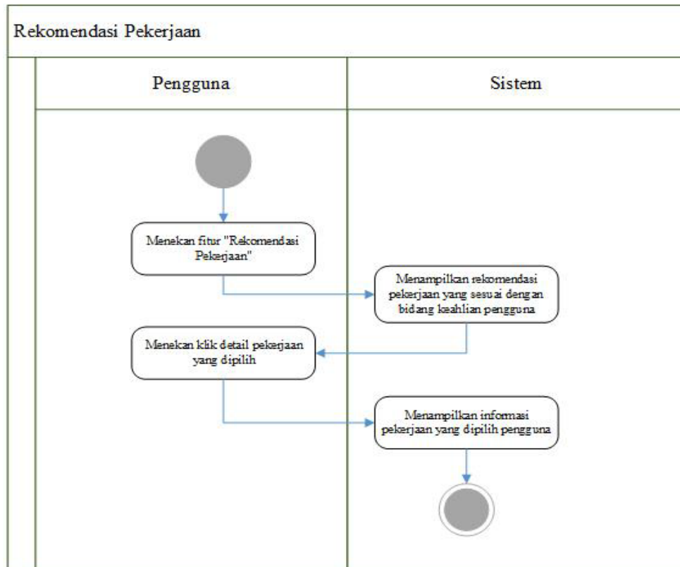
Gambar 3 Rekomendasi Pekerjaan
