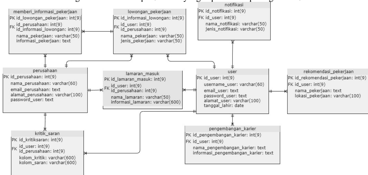
Gambar 6 Rancangan Database
