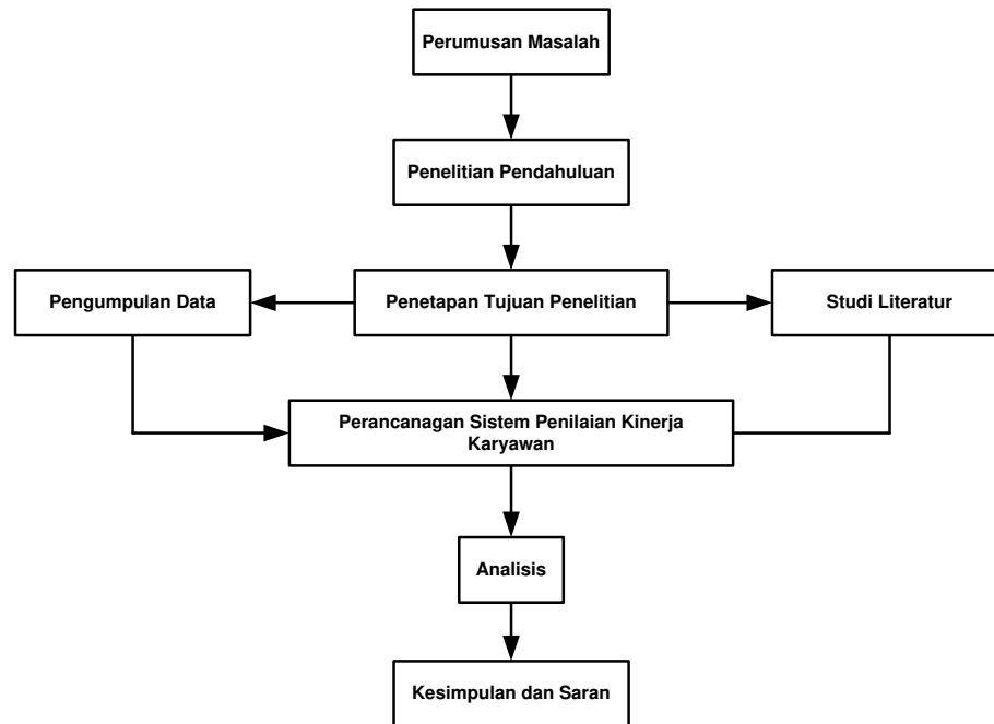
Gambar 2. Metodologi Penelitian
