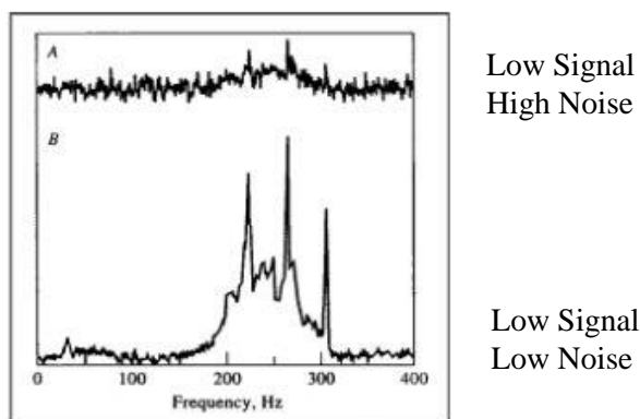
Gambar 1. Spektra Sinyal
