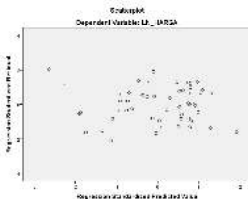
Gambar 4. Pengujian Heteroskedastisitas Setelah Transformasi Data
