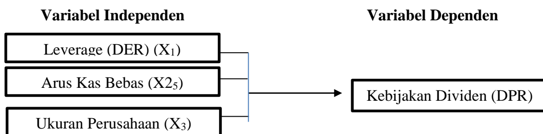
Gambar 1 Kerangka Konseptual
